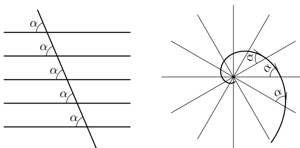
Рис. 8. Полет насекомого — по прямой и по спирали. Источник: Христо Бояджиев [1].
