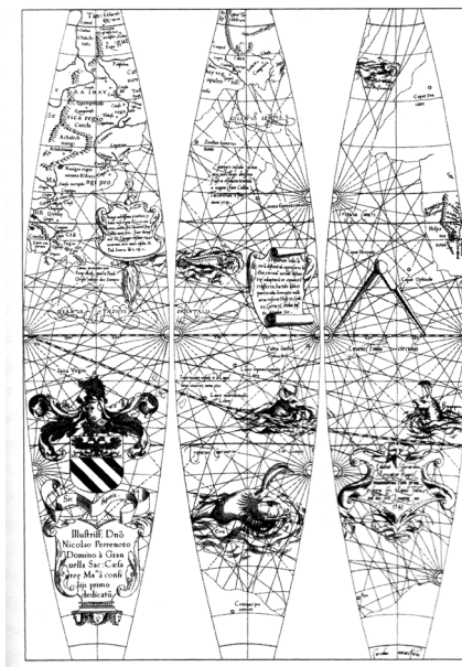
Рис. 12. Сегменты глобуса 1541 года
