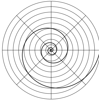
Рис. 7. Логарифмическая спираль
