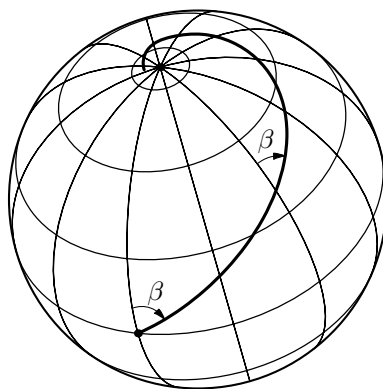
Рис. 1. Локсодрома
