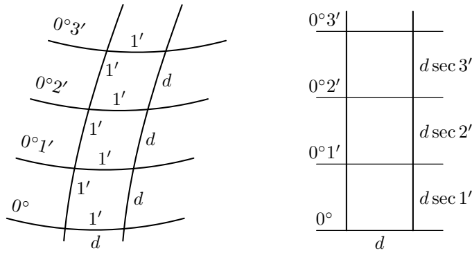
Рис. 14. Метод Райта: накапливающаяся поправка
