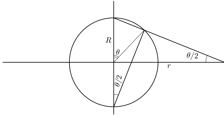
Рис. 6. Стереографическая проекция: формула (5)
