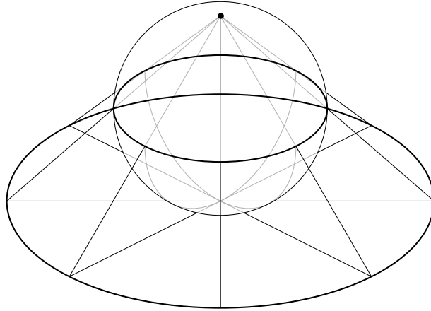
Рис. 5. Стереографическая проекция
