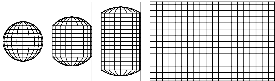
Рис. 15. Эдвард Райт: проекция Меркатора как отпечаток надувающегося пузыря. Источник: R. Israel [5]
