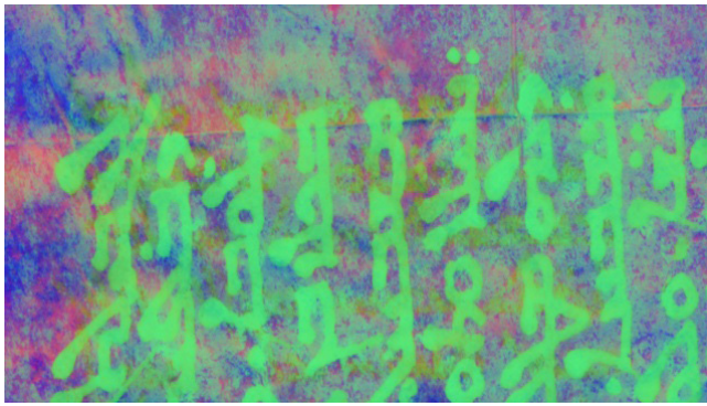
Fig. 2r: HLLE.
