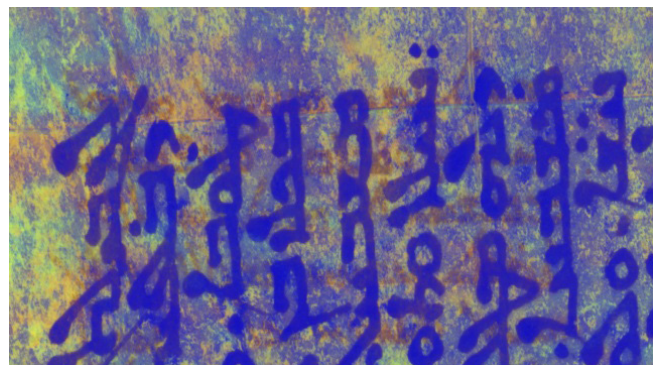
Fig. 2p: TSNE2.
